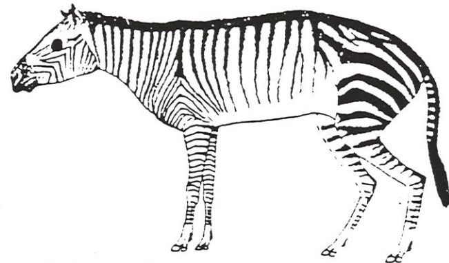
Morgenrötlerpferdchen (Eohippus). Rekonstruktion des vor ca 70 Mill. Jahren lebenden, nur 40 cm hohen Vorfahren des Einmeters.
