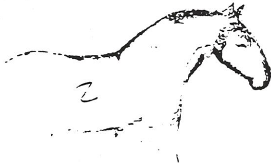
Altsteinzeitliches Höhlenbild eines südiberischen Steppensperdes der Höhle La Pileta. Prov. Málaga, Spanien (Zeichnung nach O)
